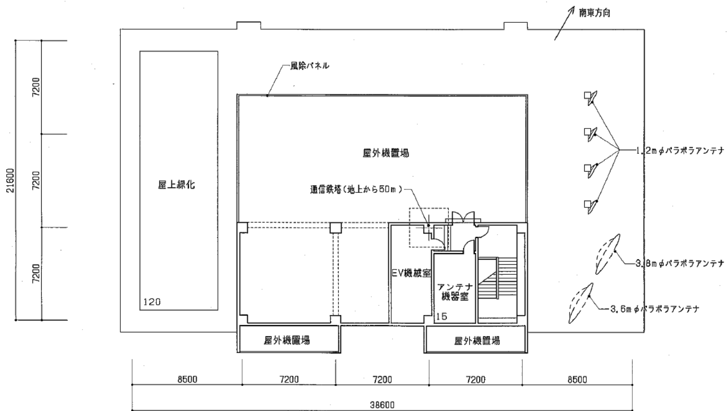
R階平面図
