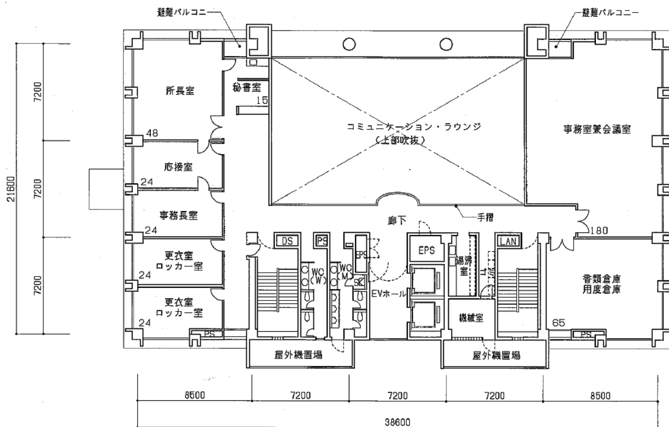
2階平面図
