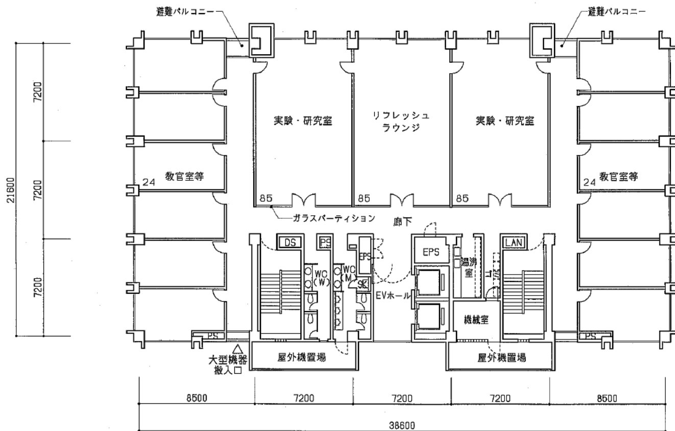
6階平面図
