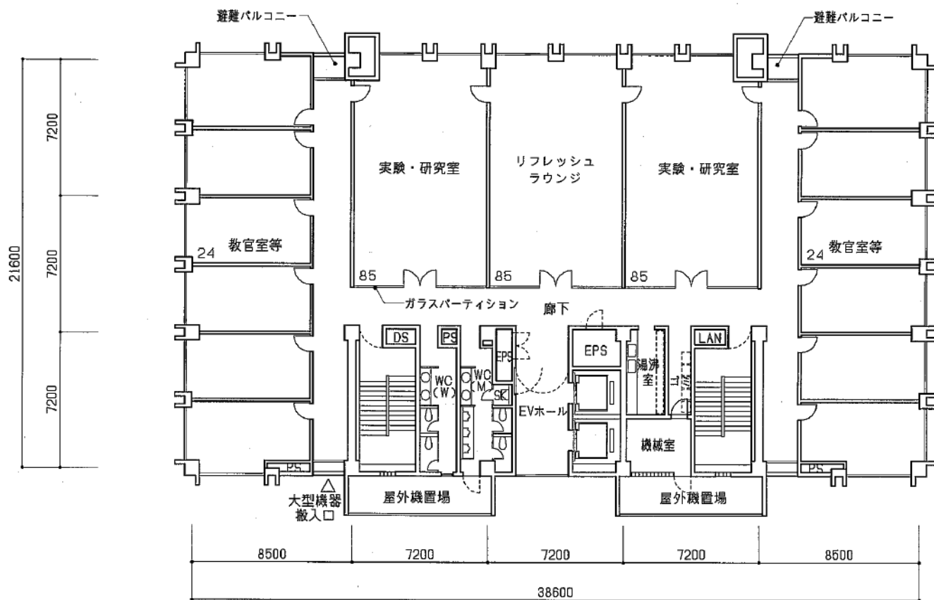
5階平面図
