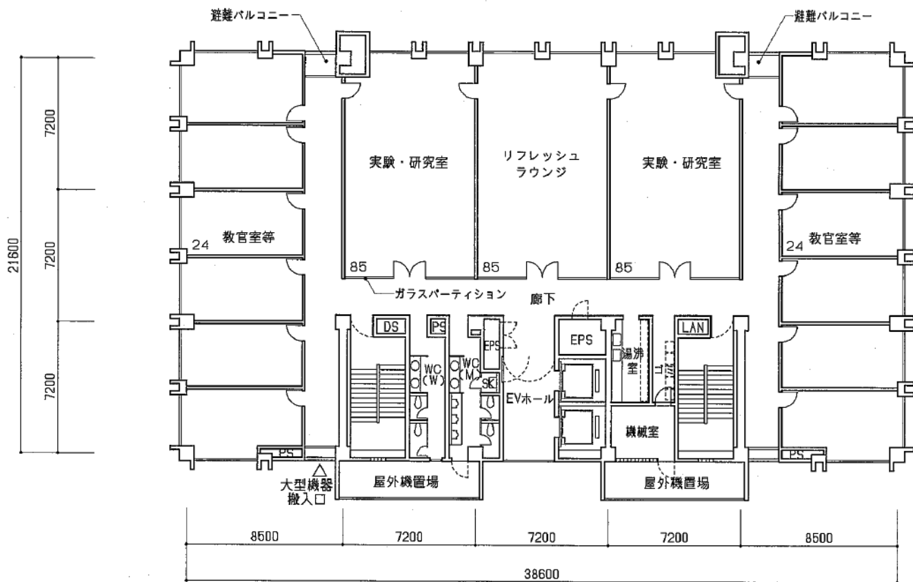
4階平面図
