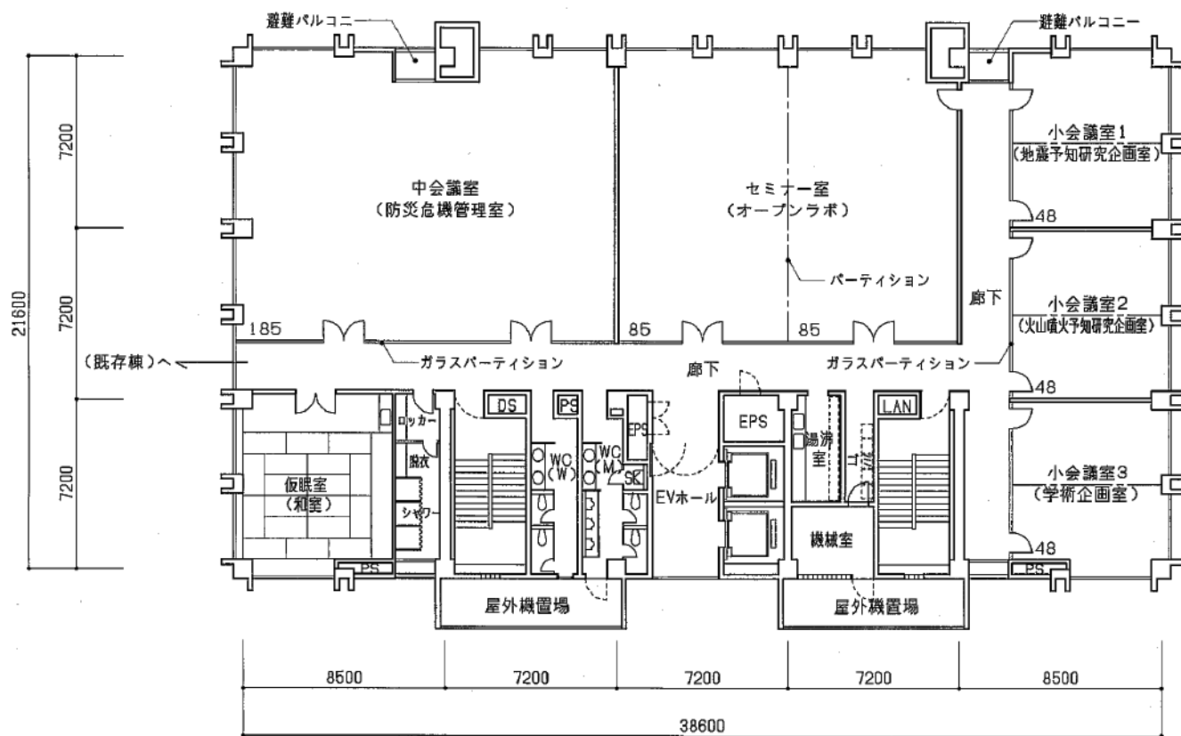
3階平面図
