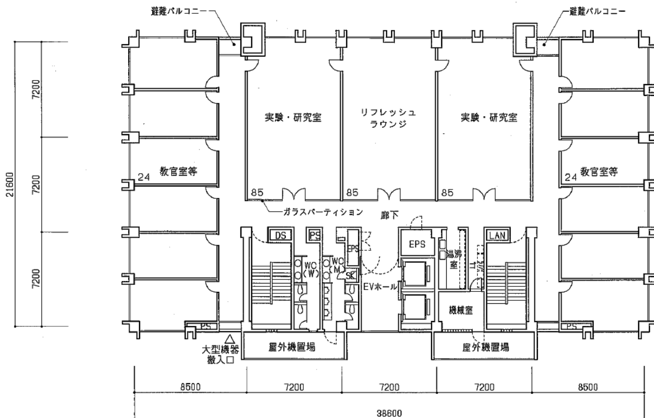
7階平面図
