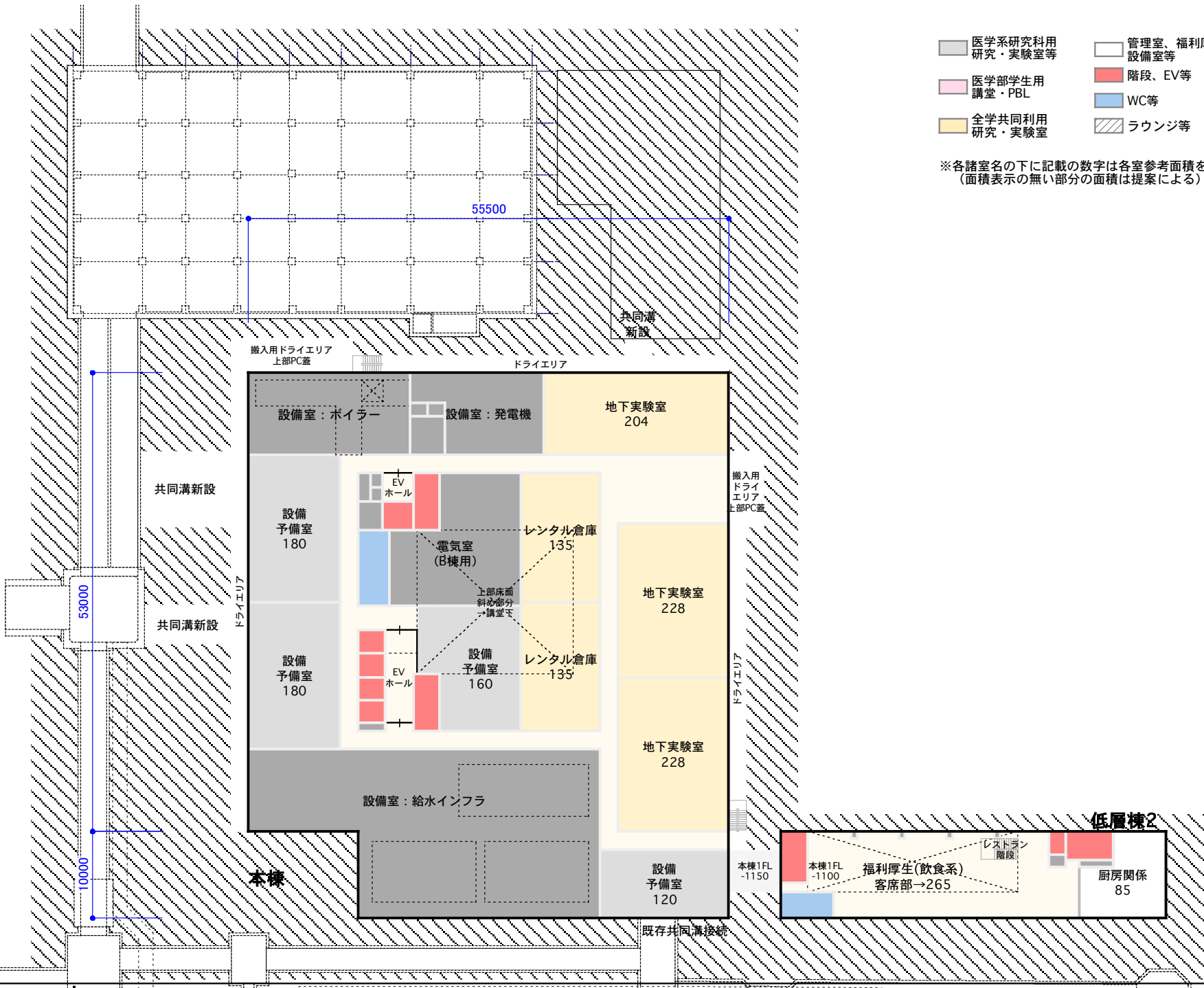
資料 17-2-2 | 参考平面図 (B棟) 地下1階
